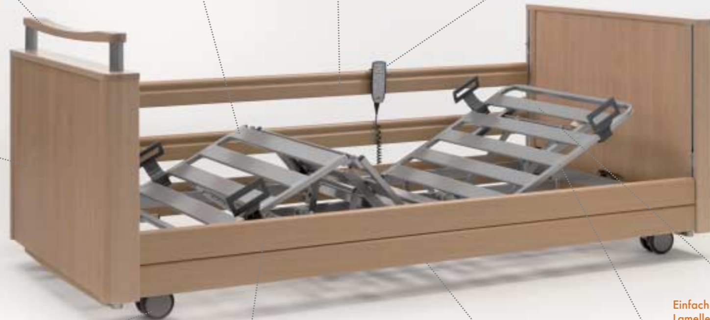
24 Volt-Antriebssystem mit selektiv-sperrbarem Handschalter
